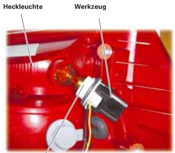
Lampenfassung
